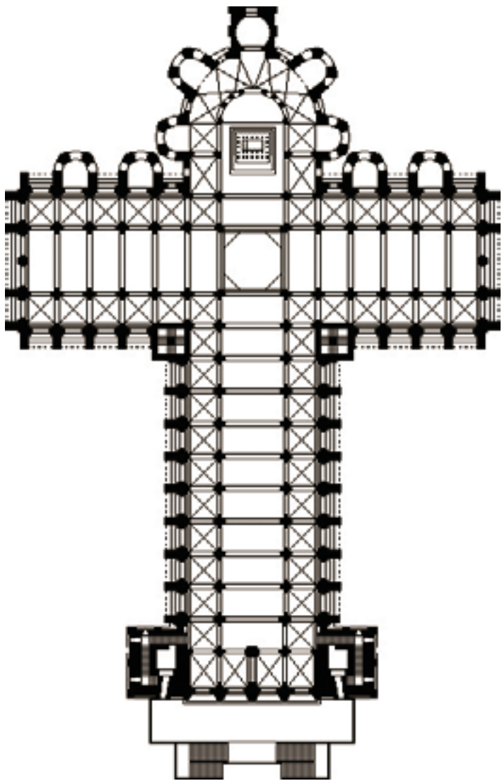
Fig. 136 PLANTA DE CREU LLATINA
