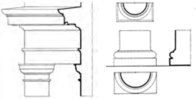
Fig. 119 ORDRE JÒNIC
