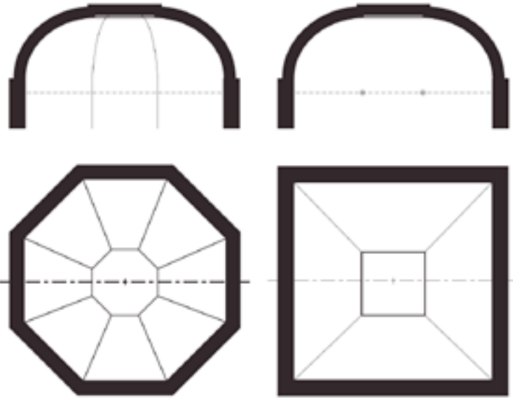
Fig. 161 VOLTES DE MIRALL
