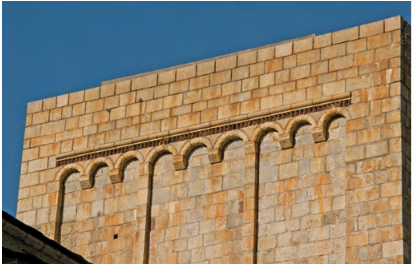
Fig. 37 BANDES LLOMBARDES
